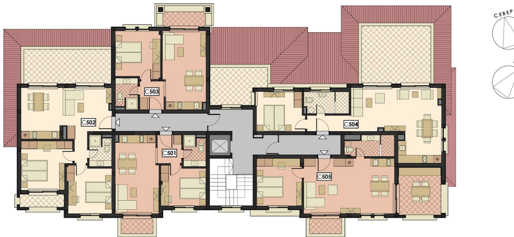
СТРАДА 03 · РАЗПРЕДЕЛЕНИЕ ПЕТИ ЕТАЖ
