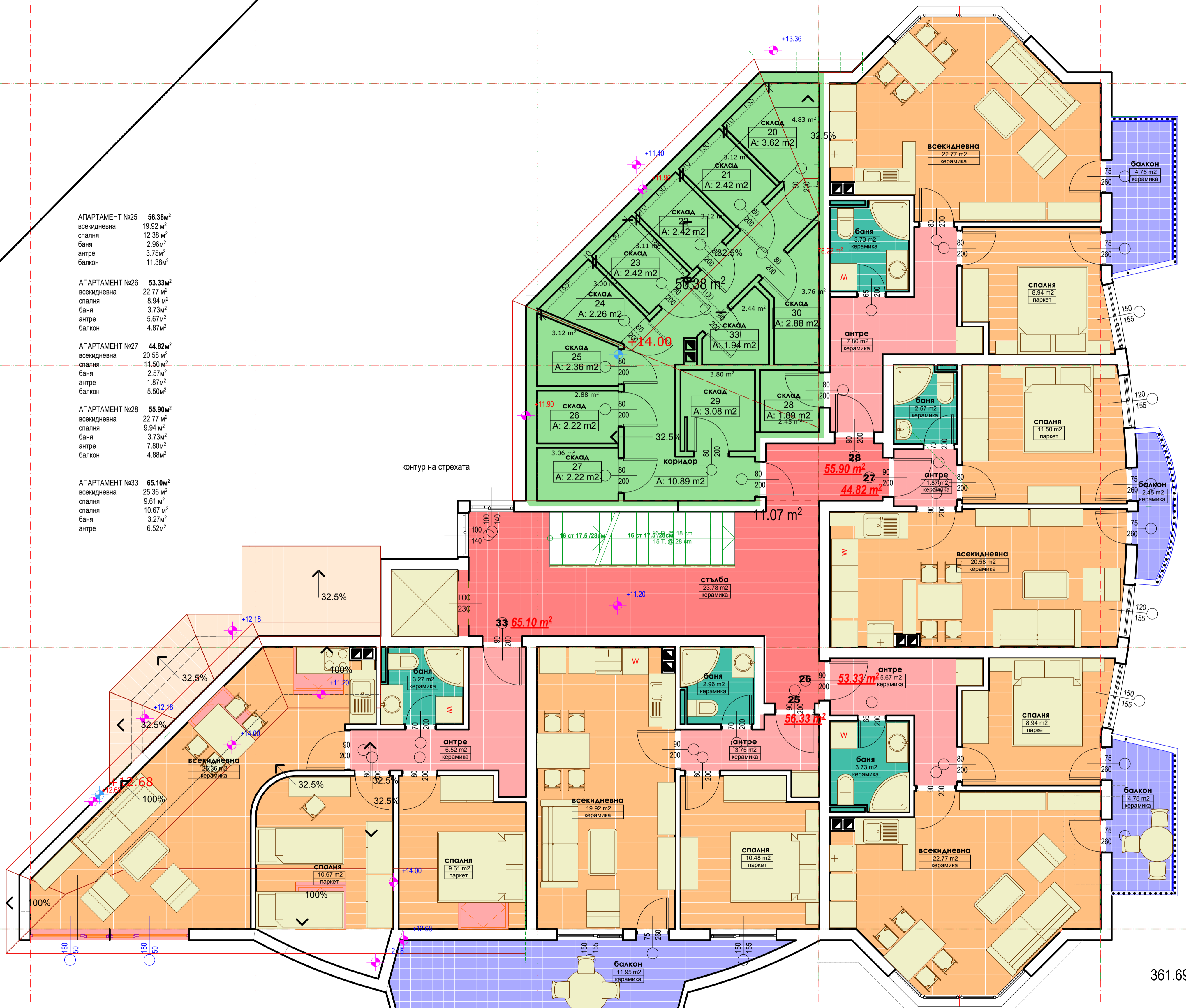
План на кота +11.20 четвърти жилищен етаж Покривни линии М 1: 50
